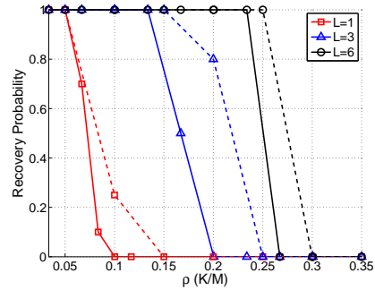
(d) Probability of recovery, \delta = 1.2
