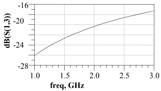
Figure 11.b : Isolation égale à -21 dB à la fréquence RF de l'ordre de 1,9 GHz pour Z_0 = 50 \Omega
