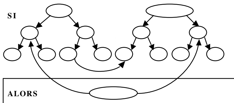
FIG. 3 — Une règle sur un graphe RDF.
