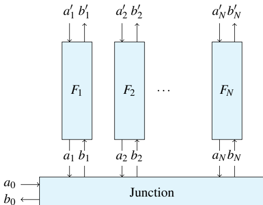
Fig. 1. Multiplexer
