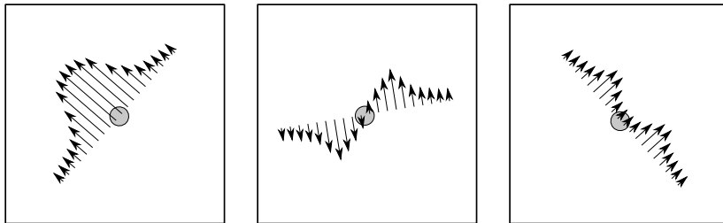
Fig. 1. A 0 th -order jet Fig. 2. A 1 st -order jet Fig. 3. A 2 nd -order jet
