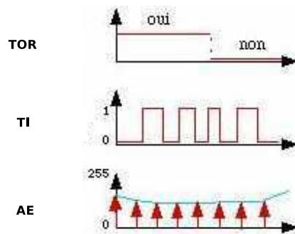
Figure 3.4 — Différentes formes des signaux des capteurs considérés.
