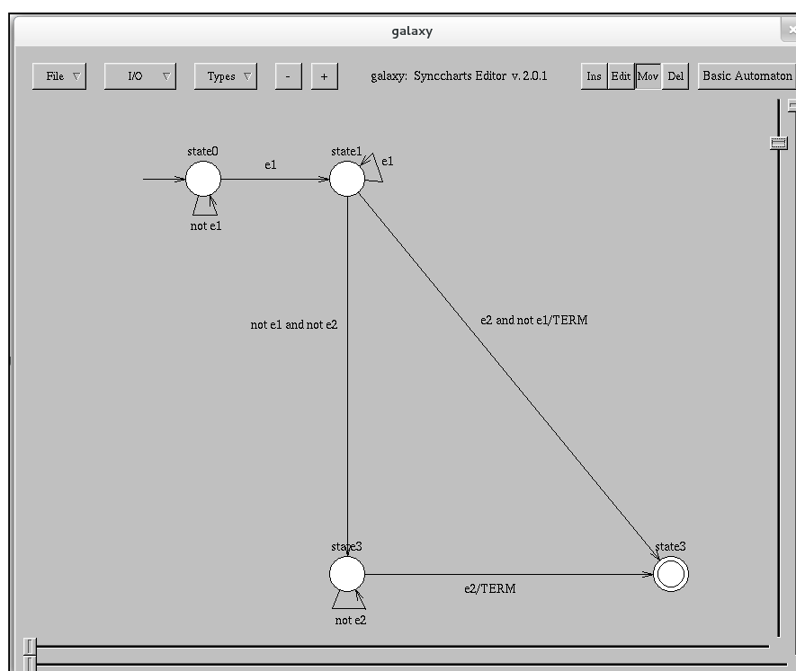
Figure 4.2 — Édition du modèle e1 Before e2 en utilisant l'outil Galaxy.
