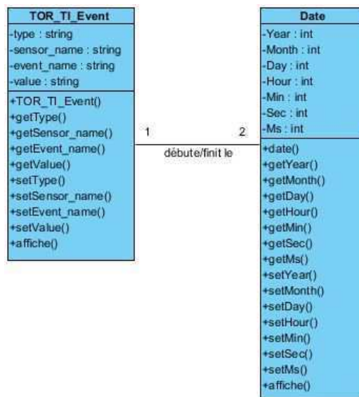
Figure 3.8 — Classe TOR_TI_Event des événements des capteurs de type TOR ou TI.
