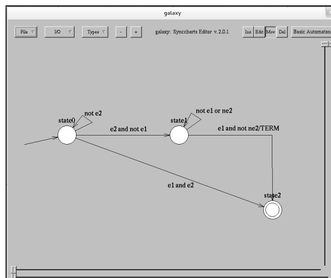
Figure 4.6 — Édition du modèle e1 Overlaps e2 en utilisant l'outil Galaxy.
