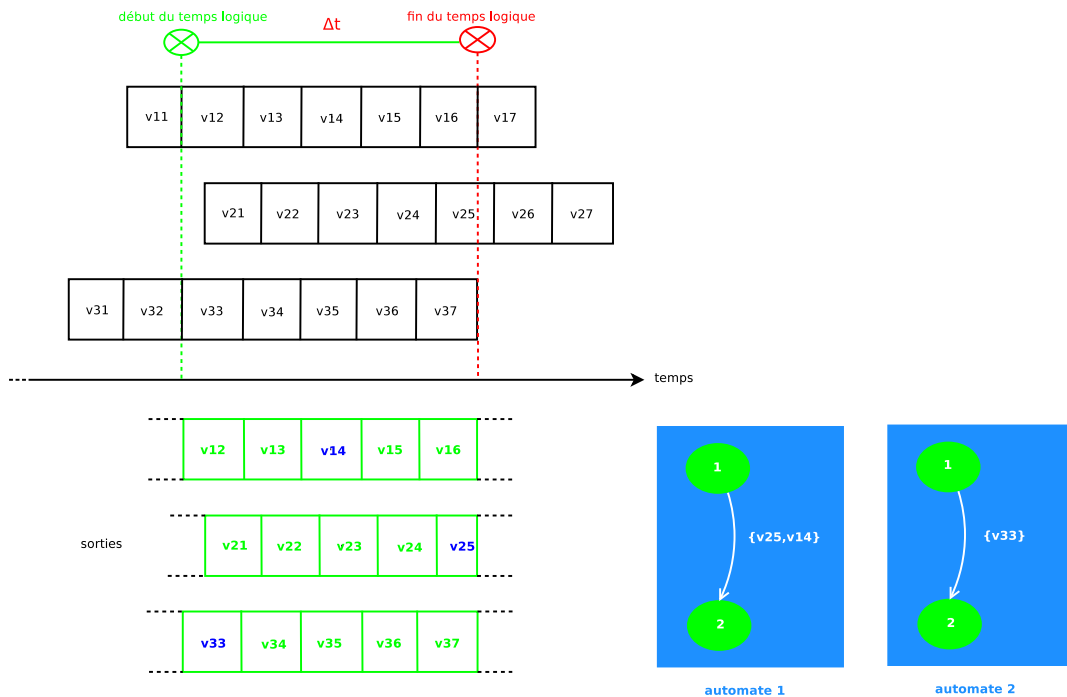
Figure 3.13 — Résultat du fonctionnement de la machine d'exécution dans le cas normal : Définition standard de l'instant logique.
