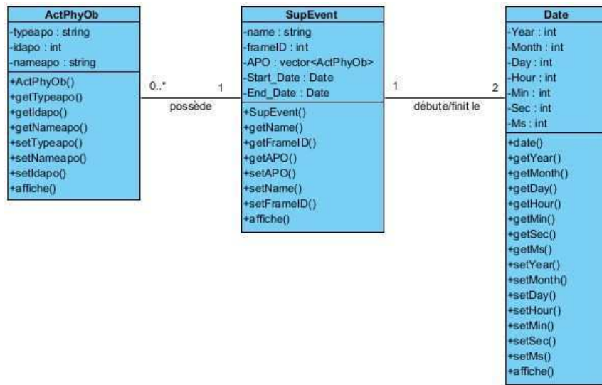
Figure 3.7 — Classe "SupEvent" des événements vidéo de la plate-forme SUP.
