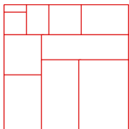
(d) ROTreeMapLayout
