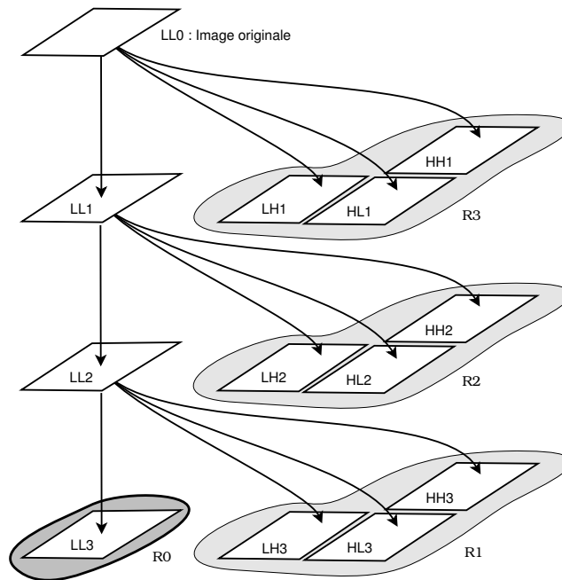
Figure 4.8. Regroupement des sous-bandes en niveaux de résolution ( D=3 )
