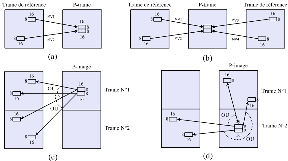
Figure 6.12. Prédiction 16 \times 8 : (a) pour une P-trame, (b) pour une B-trame, (c) pour la trame n°1 d'une P-image, (d) pour la trame n°2 d'une P-image
