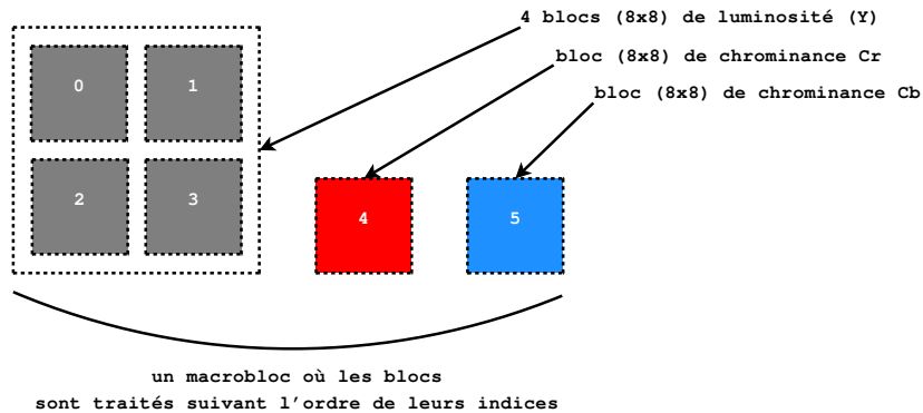
Figure 5.5. Définition d'un macrobloc
