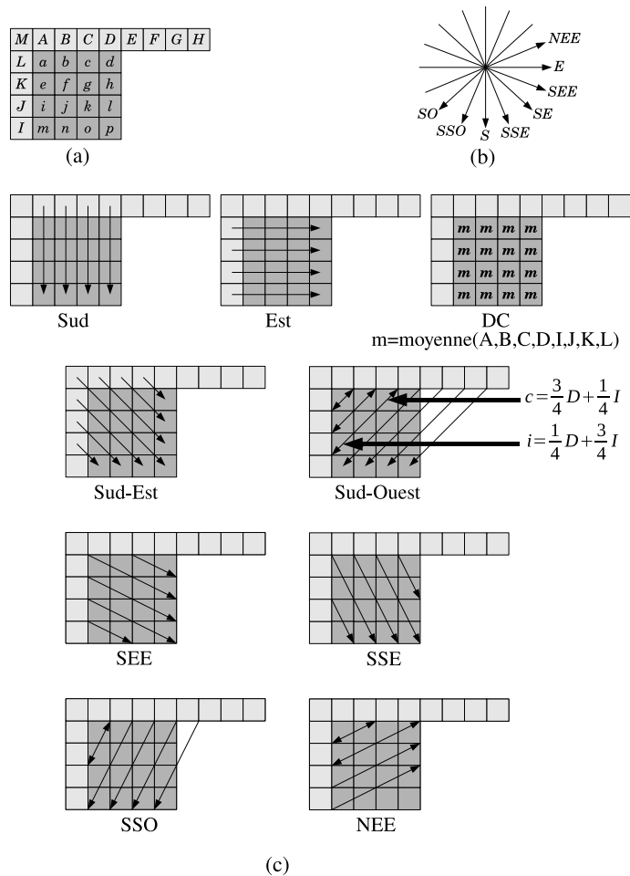
Figure 7.34. Les neuf options de prédiction du mode Intra_4 × 4
