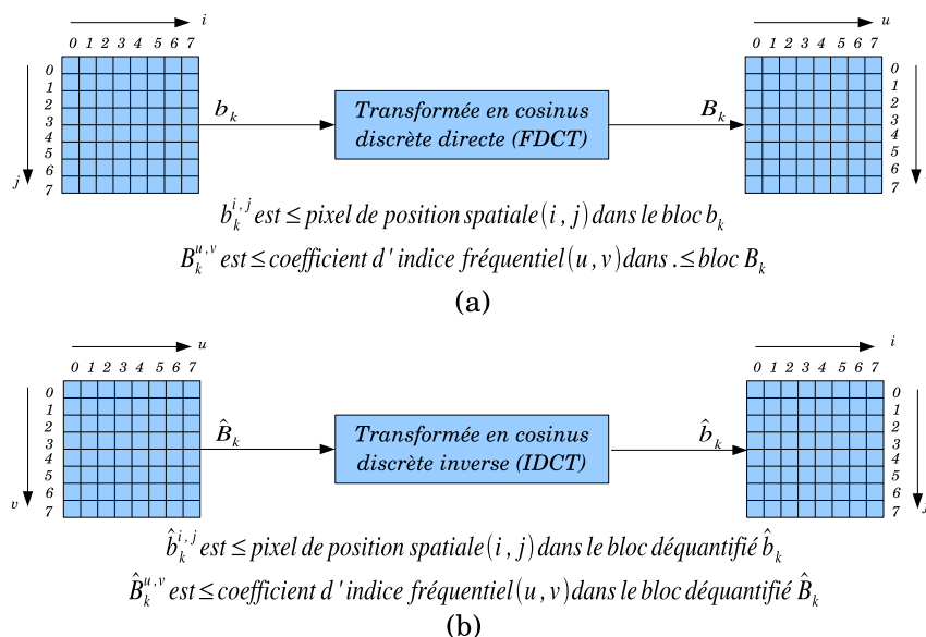
Figure 3.5. Analyse spectrale d'un bloc : (a) transformée directe du codeur et (b) transformée inverse du décodeur
