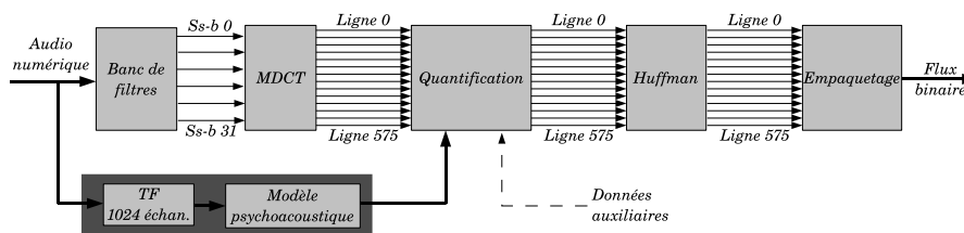
Figure 5.14. Principe de la couche III
