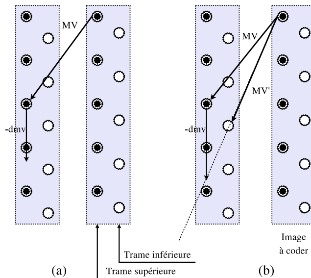
Figure 6.13. Prédiction dual prime : (a) le vecteur MV indique le déplacement entre les macroblochs des trames de même parité ; (b) Le vecteur différentiel, dmv , permet de reconstruire le vecteur MV' , associé à la trame de parité inverse
