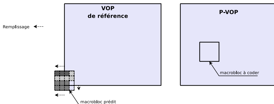
Figure 7.10. Remplissage des pixels du macrobloccs se situant au-delà des limites du VOP
