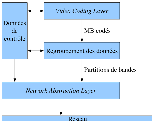
Figure 7.28. Séparation du codage en une partie VLC et une partie NAL
