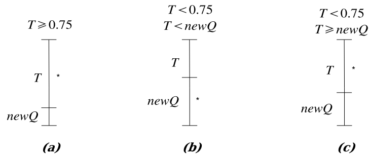
Figure B.7. Le fonctionnement de la fonction Codage_MPS() : l'intervalle sélectionné est marqué d'un astérisque
