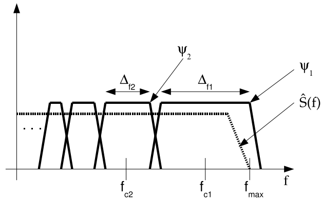
Figure 2.23. Le recouvrement par les ondelettes peut s'identifier à une analyse par un banc de filtres à Q -constant
