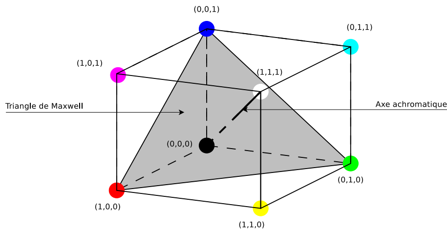
Figure 4.11. L'espace CIE RGB
