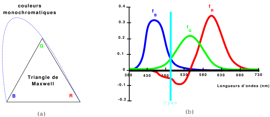
Figure 4.10. (a) Définition des couleurs monochromatiques par rapport au triangle de Maxwell. (b) Fonctions colorimétriques des primaires R, G et B.
