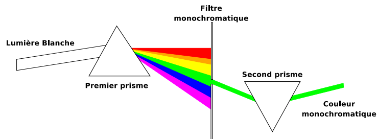
Figure 4.7. L'expérience d'Isaac Newton
