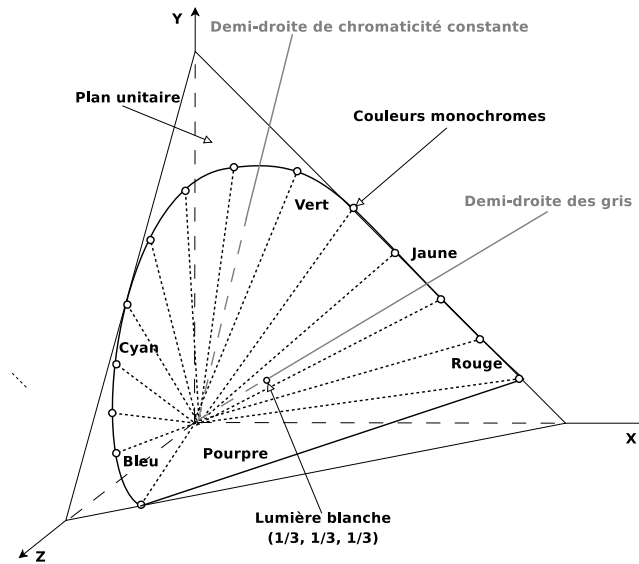
Figure 4.14. Toutes les couleurs sont définies dans le premier octant de l'espace tridimensionnel CIE XYZ
