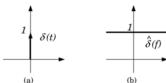
Figure 3.6. (a) L'impulsion de Dirac \delta(t) , et (b) sa représentation fréquentielle \hat{\delta}(f)
