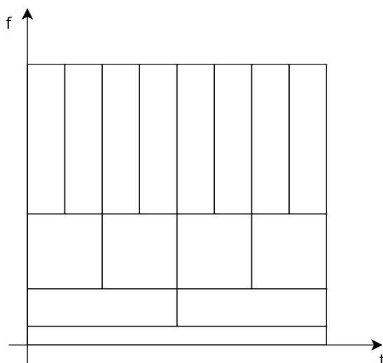
Figure 2.20. Pavage adaptatif respectant le principe d'incertitude
