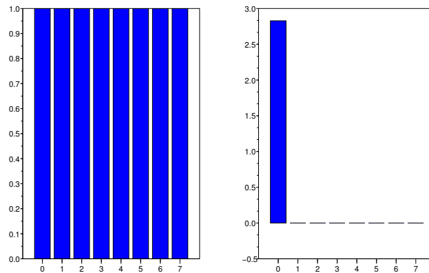
Figure 2.12. Le graphe de gauche montre un signal carré : s[k] = 1(0 \leq k < 8) , celui de droite sa DCT ID
