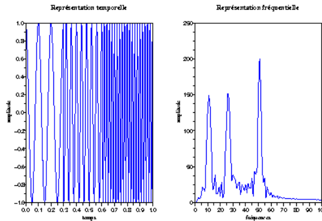
Figure 2.16. Les représentations temporelle et spectrale du signal s_2(t)
