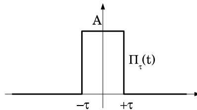
Figure 3.4. Le signal rectangulaire \Pi_\tau(t)
