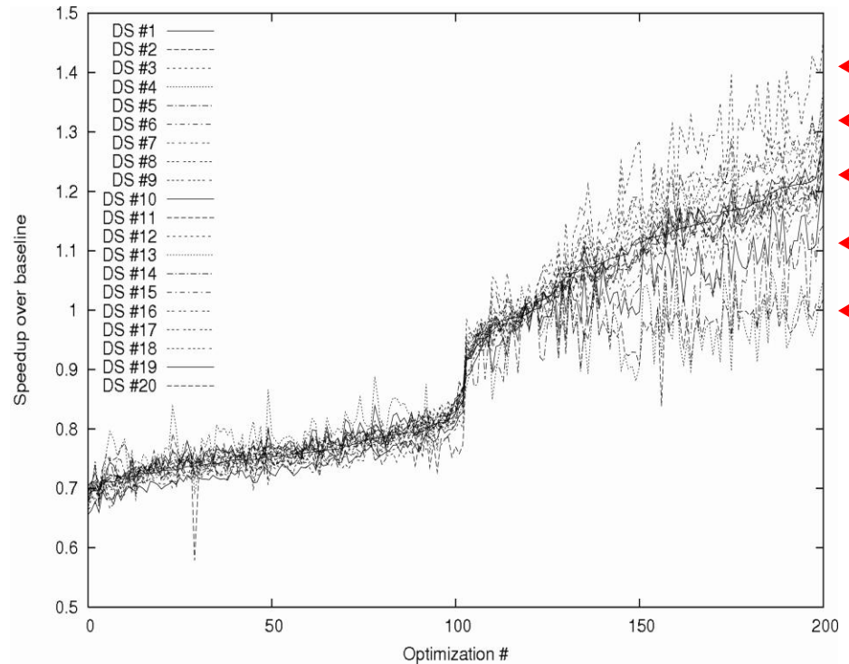
jpeg_d (clustering)
