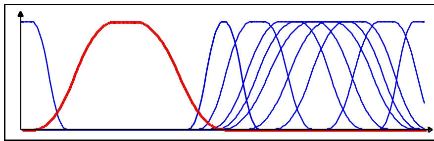
Figure 19 : Solutions de la forme \zeta m_\beta P \hat{E} avec \rho^* = 0.3
