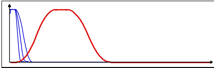
Figure 18 : Solutions de la forme \zeta f_x m_\beta A \hat{E} avec \rho^* = 0.3
