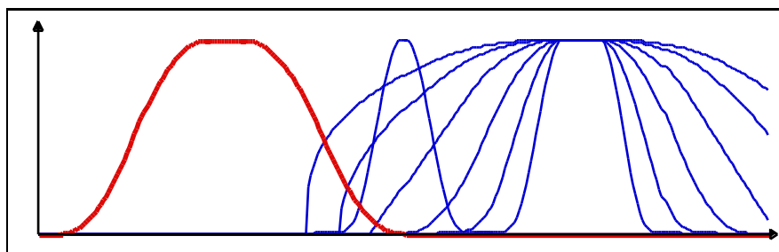
Figure 20 : Solutions de la forme \zeta f_x P \hat{E} avec \rho^* = 0.3
