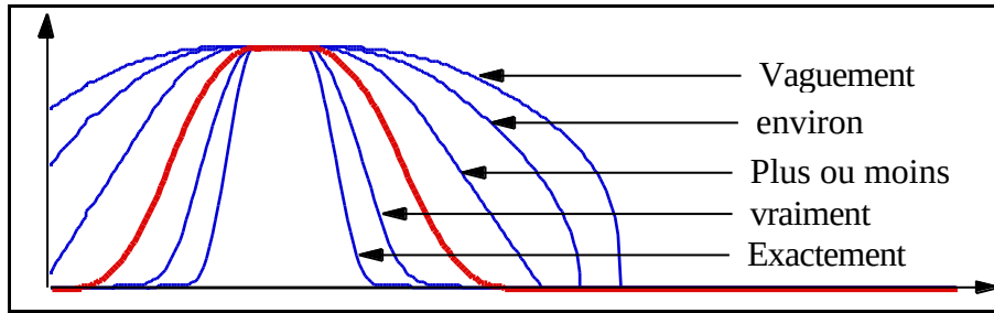
Figure 6. Opérateurs flous appliqués à la propriété simple \zeta^- \text{important} \hat{E}
