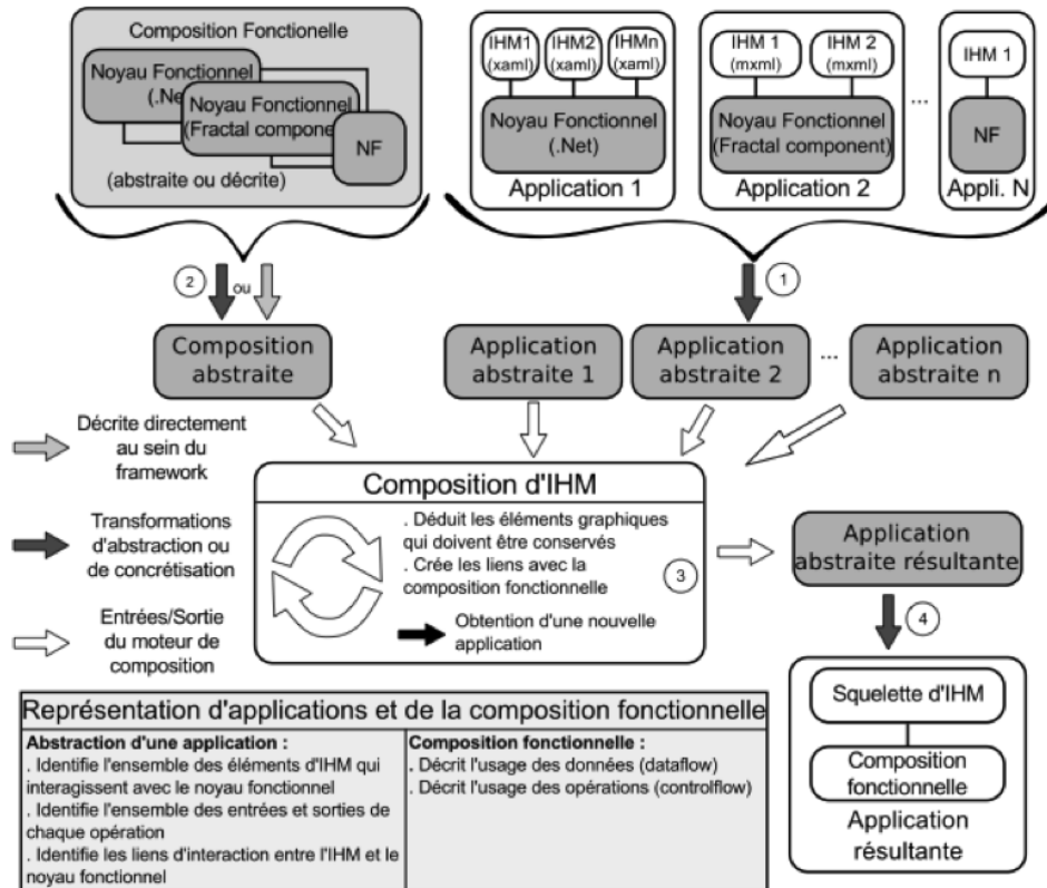
Figure 5. Démarche globale pour la réalisation de la composition d'applications proposée dans [JOF 11]
