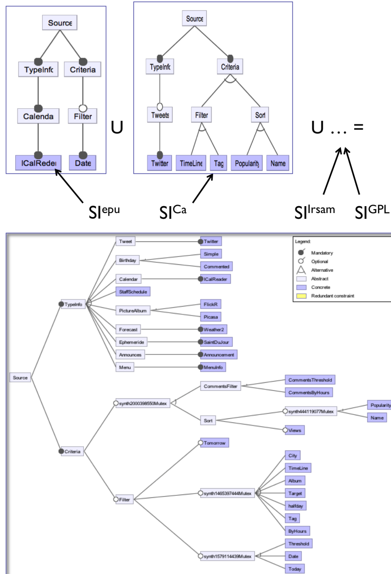
Figure 3. Capture de la variabilité par "feature models". Deux FM sont visualisés à gauche, ils sont extraits de systèmes pré-existants dans le cadre du projet YourCast http://yourcast.fr . Le premier présente une source d'information diffusant des calendriers qu'il est possible de trier par date. La seconde diffuse des tweets. Ceux-ci peuvent être triés ou filtrés. L'analyse d'un ensemble de tels systèmes a conduit à la modélisation de différents FM, fusionnés à droite pour modéliser la variabilité des sources d'informations disponibles.
