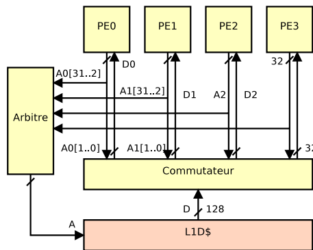
Figure 4. Diagramme de l'unité de lecture mémoire d'une architecture SIMT
