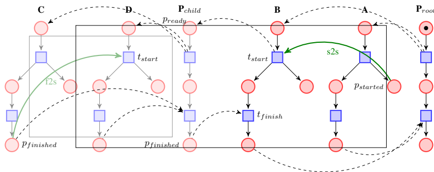
Figure 5. Réseau de Petri résultant de la transformation
