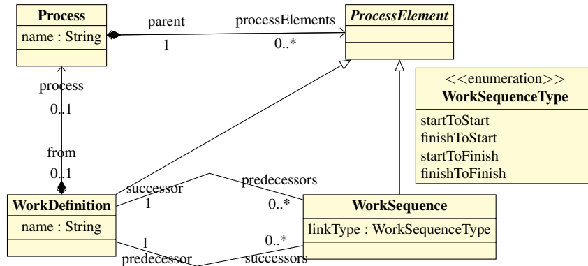
Figure 2. Métamodèle SimplePDL
