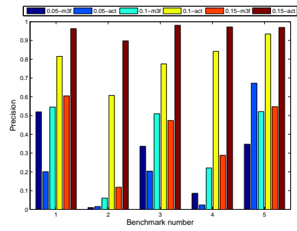
(b) Precision
