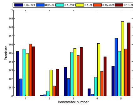
(b) Precision
