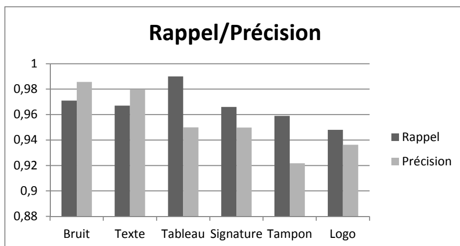
Figure XI. Résultat de la classification pour les 6 types de zones.
