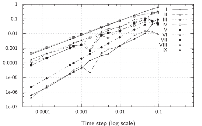
(d) The linear oscillator (Example 2). Coordinate error
