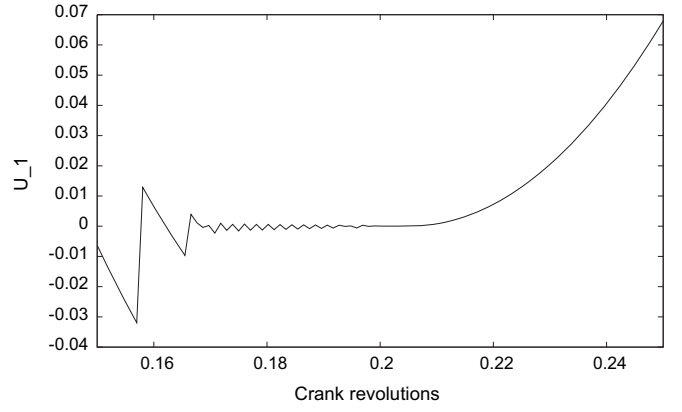
(d) Direct projected scheme (Algorithm 1) on [0.15, 0.25] .
