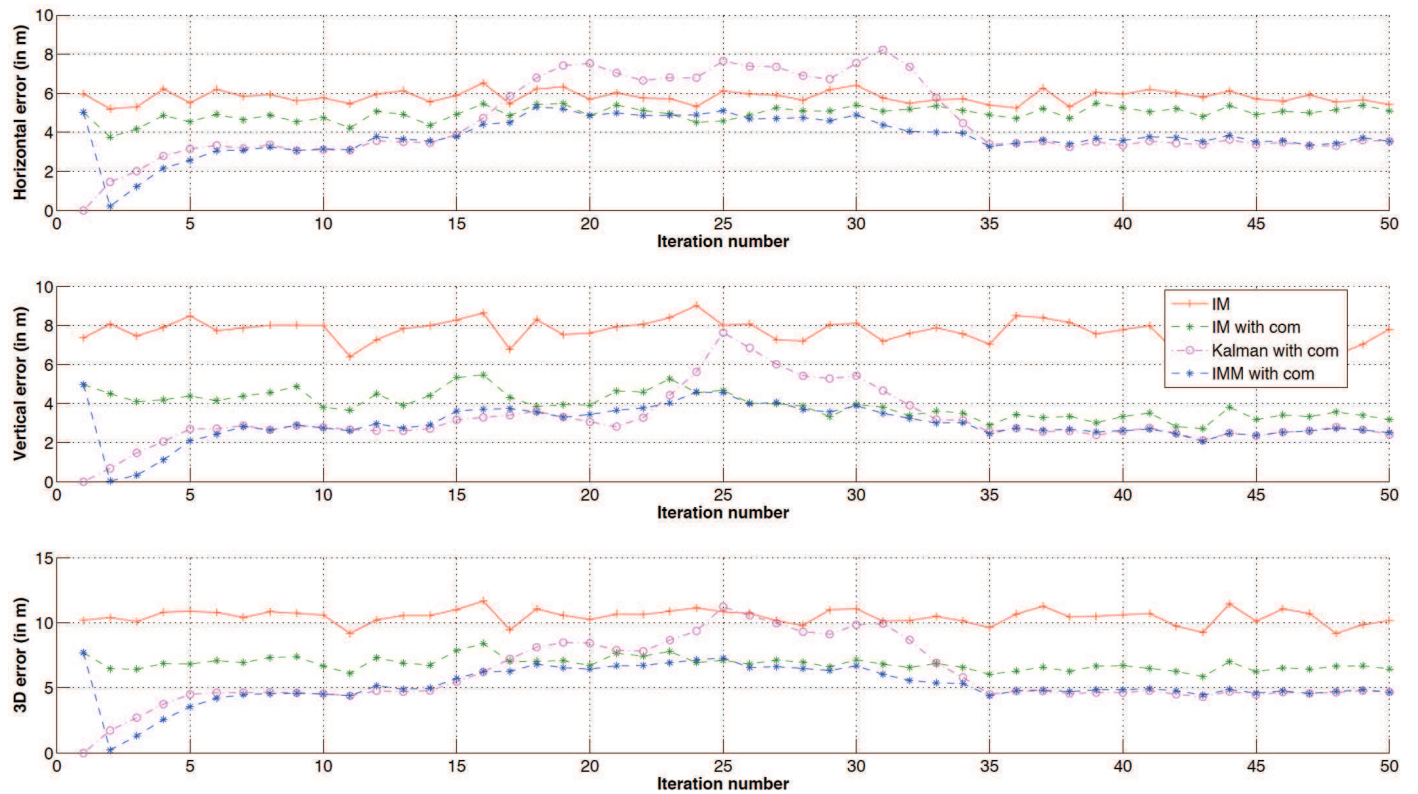
Figure 7. Positionning error
