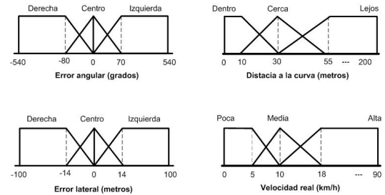
Figura 3: Funciones de pertenencia para el control del volante en rectas y curvas
