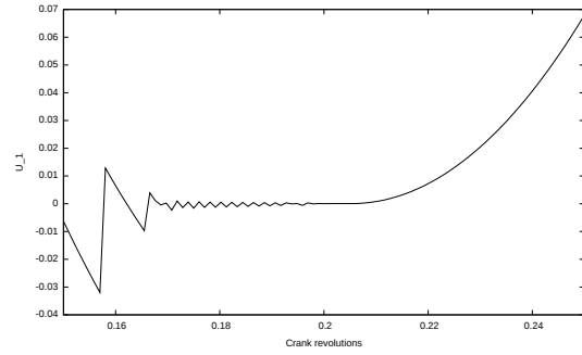
(d) Direct projected scheme (Algorithm 1) on [0.15, 0.25] .
