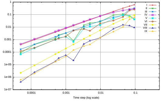
(d) The linear oscillator (Example 2). Coordinate error
