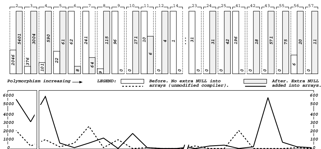
Figure 9: Propagation du type NULL des tableaux vers les variables locales. Mesures avant et après infection artificielle.
