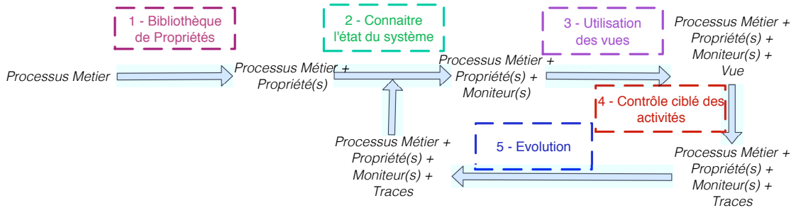
FIGURE 1. L'approche SMILE
