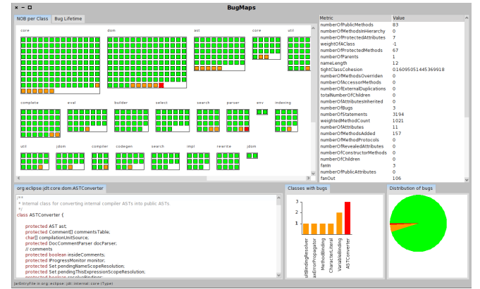
Fig. 3. BugMaps: snapshot browser
