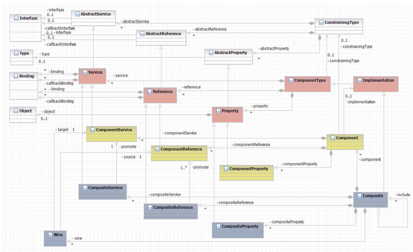
Figure C-2. SCA meta-model.
