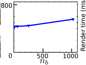
n_b = 1024
