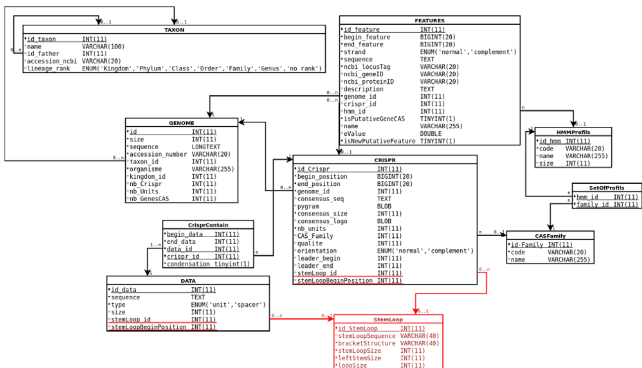
figure 7: Nouveau schéma de la base de données CRISPR
