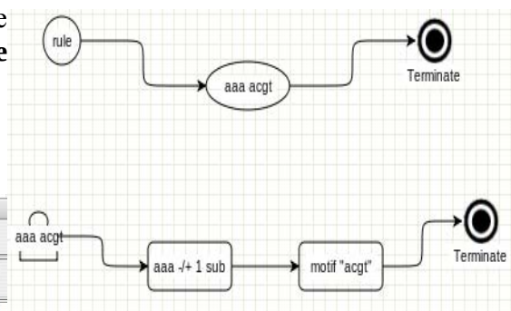
figure 9: Modèle Logol graphique
