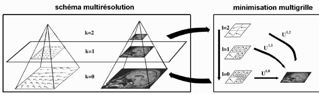
FIG. 3 – Exemple de relaxation multigrille à une résolution donnée. À chaque niveau de résolution (à gauche), une stratégie multigrille (à droite) est mise en place. Pour des raisons de clarté, le fonctionnement tridimensionnel de la méthode est ici illustré en 2D.
